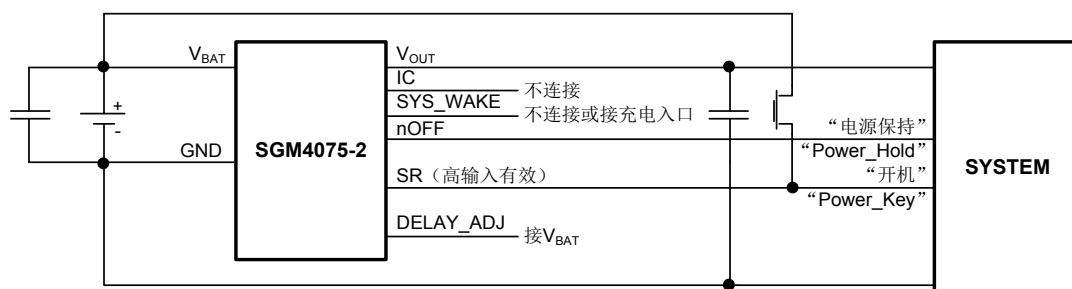
图 1. 采用惯用“开机”和“电源保持”2个控制信号的应用电路
