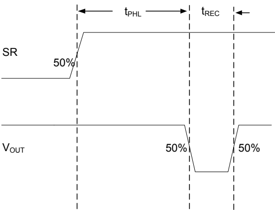
图 8. RESET Timing 1
