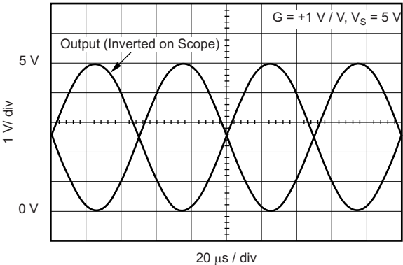
图 24. OPA348 具有 轨至轨输入和输出
