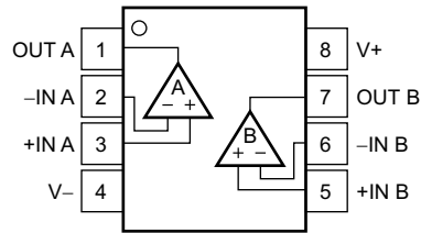
引脚功能：OPA2348
