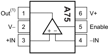
OPA373: DBV 封装 6 引脚 SOT-23 俯视图
