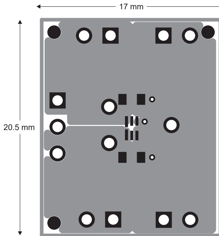
Figure 21. DSE EVM Top Layer
