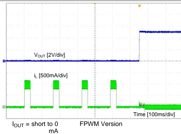
图 26. Short Recovery
