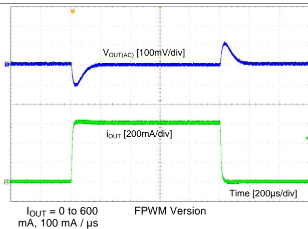
图 23. Load Transient
