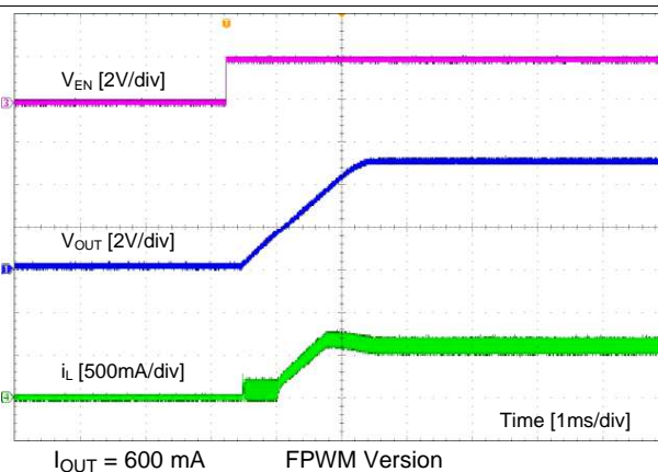
图 22. Start-Up by EN
