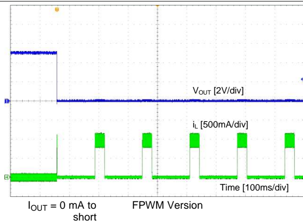
图 25. Short Protection
