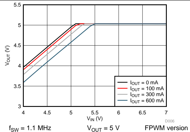
图 8. Dropout
