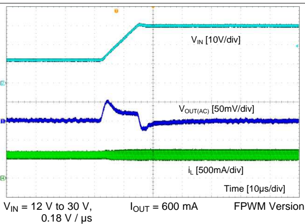
图 24. Line Transient
