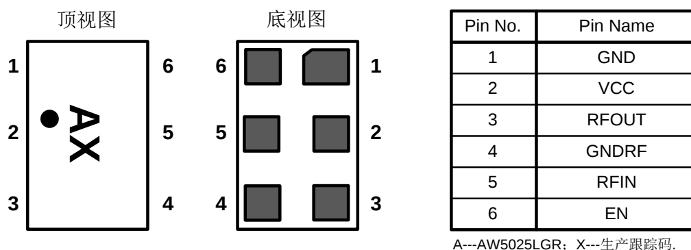
图 1. AW5025 引脚分布及标识图
