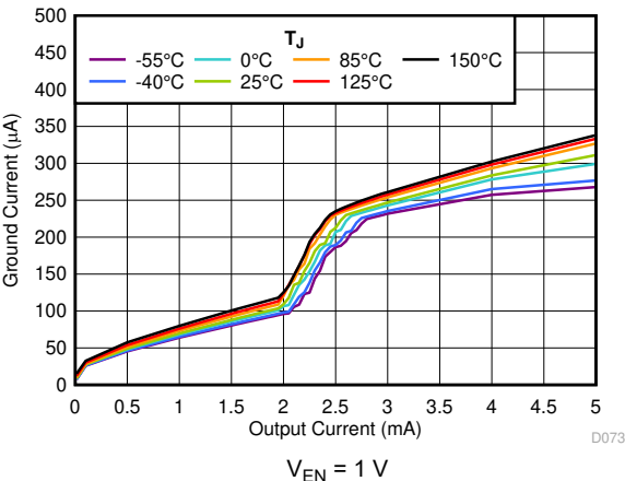
图 6-40. I_{GND} vs I_{OUT}
