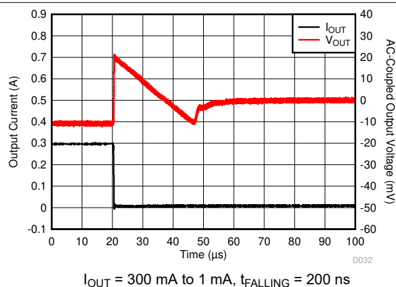
图 6-54. Load Transient
