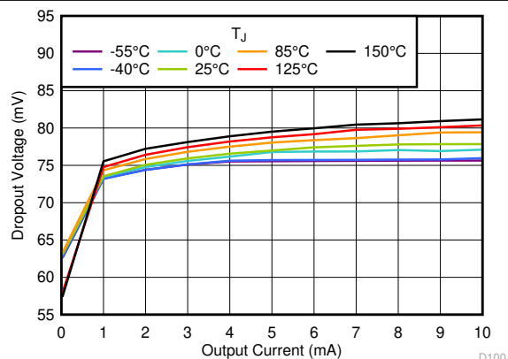
图 6-28. Dropout Voltage vs I_{OUT}
