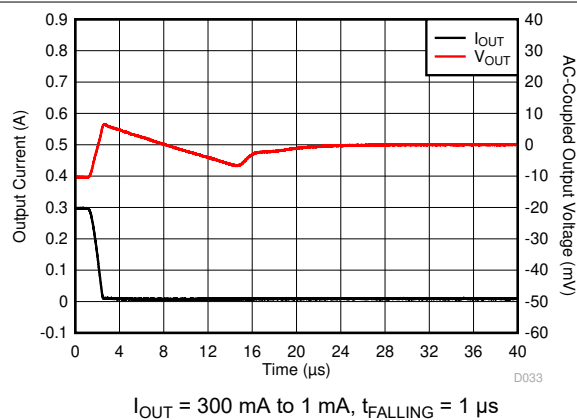
图 6-52. Load Transient
