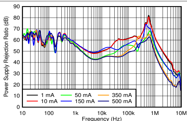
Figure 8-9. PSRR
