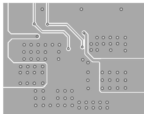
Inner Layer 2
