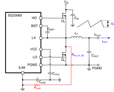
Fig 13(a). Programmable OCP Rds_on Mode
