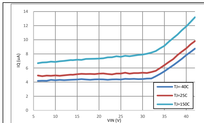
LN20542Q1, Fixed V_{OUT} = 5\text{V} , No load
