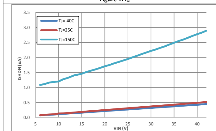
LN20442Q1, Fixed V_{OUT} = 5\text{V} , No load
