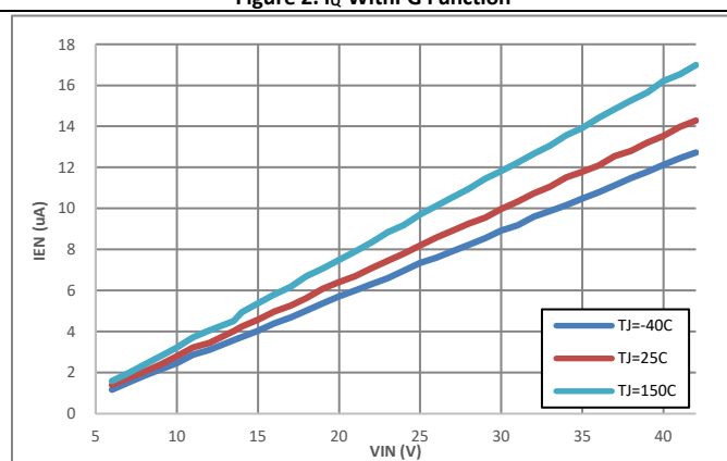
LN20442Q1, Fixed V_{OUT} = 5\text{V} , No load
