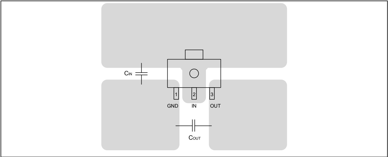
SOT89-3(ET533XXC)
