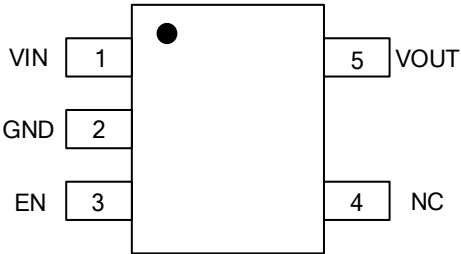
ET533XX(SOT23-5)/ ET533XXSC(SC70-5)
