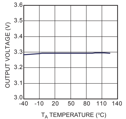
VOUT vs. TA
