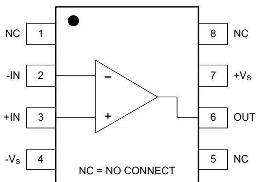
SOIC-8
