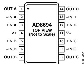
图4. 14引脚SOIC和14引脚TSSOP
