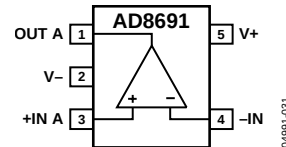
图2. 5引脚SC70
