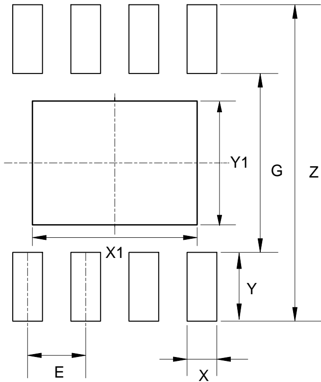
PSOP-8
