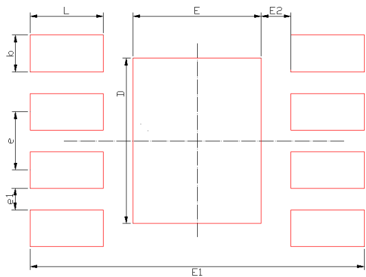
ESOP8
