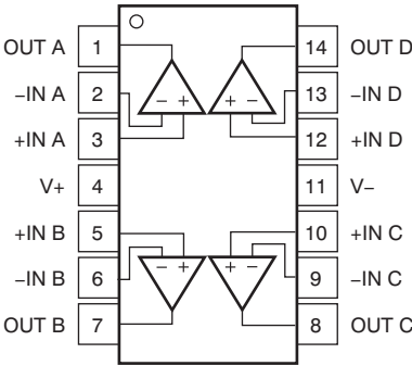
D 和 PW 封装: OPA4171 SO-14 和 TSSOP-14 (顶视图)
