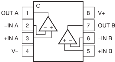
D, DCU 和 DGK 封装: OPA2171 SO-8, VSSOP-8, 和 MSOP-8 (顶视图)
