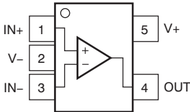
DRL 封装: OPA171 SOT-553 (顶视图)
