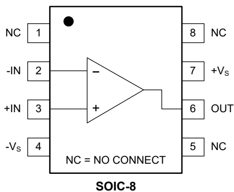
SOIC-8
