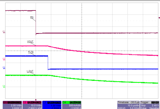
Figure 20. EN Turn OFF Delay : EN \downarrow to Fault \downarrow
