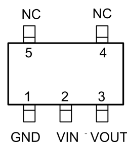
SOT-23-5L
