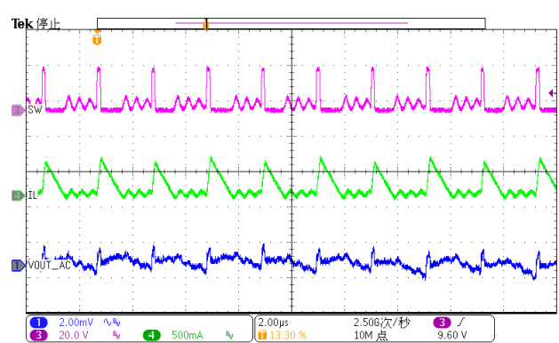
Figure 22. Output Ripple (Iload=100mA)
