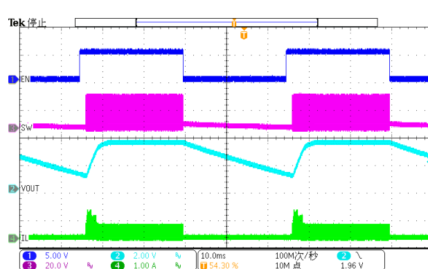
Figure 16. EN toggle (Iload=20mA)
