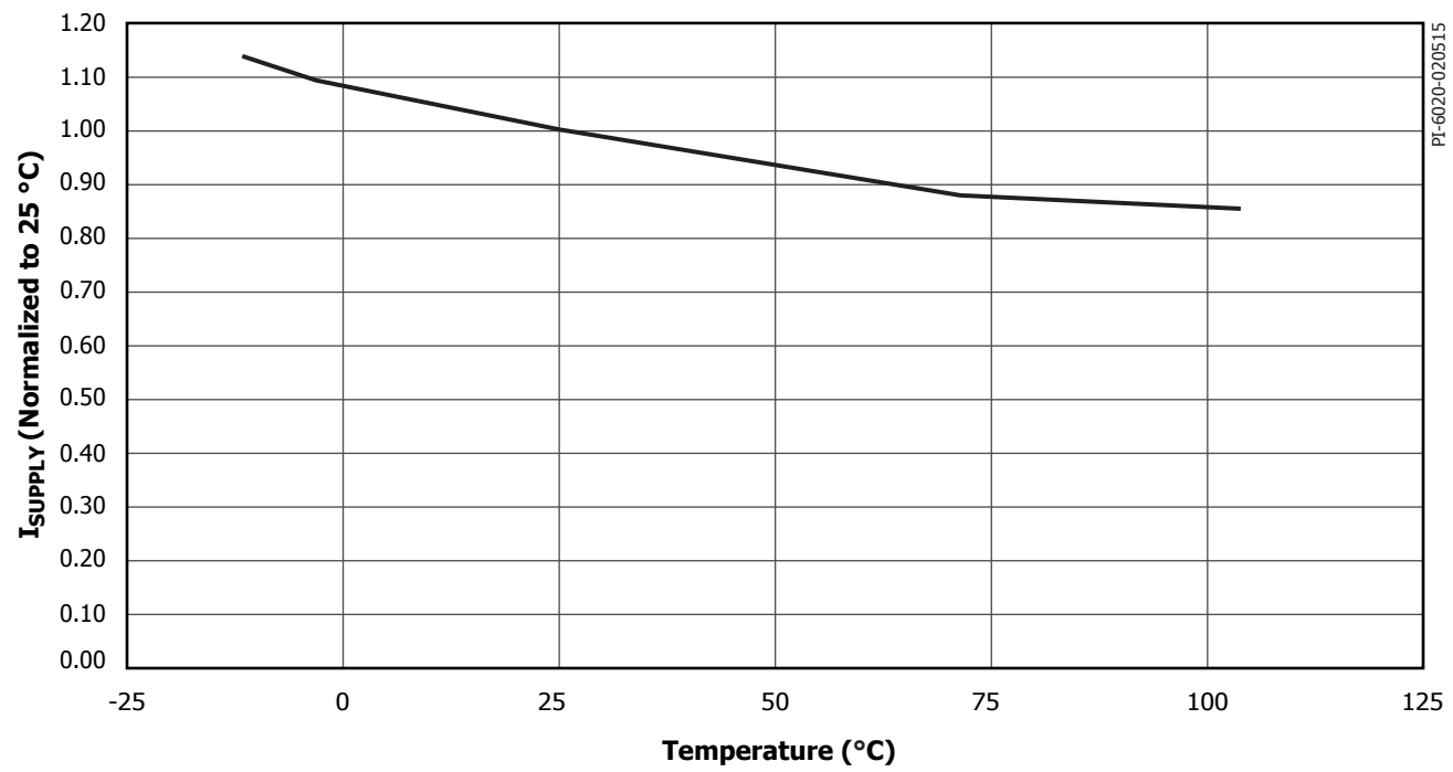
图6. I_{\text{SUPPLY}} 相对于温度的变化
