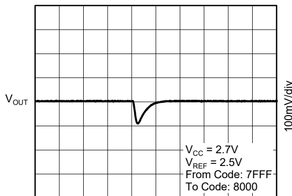
Glitch Energy: 2.7V, 1LSB Step, Rising Edge
