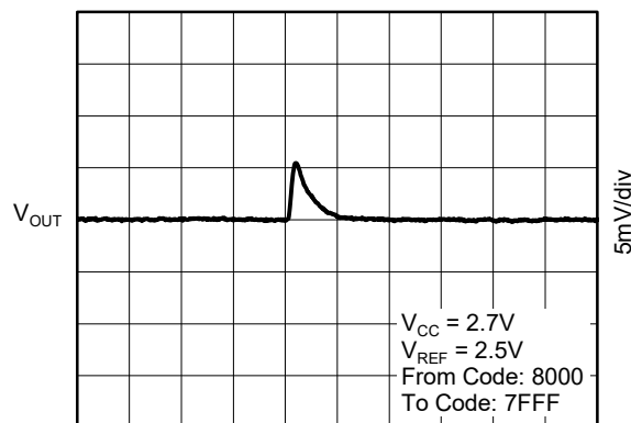
Glitch Energy: 2.7V, 1LSB Step, Falling Edge
