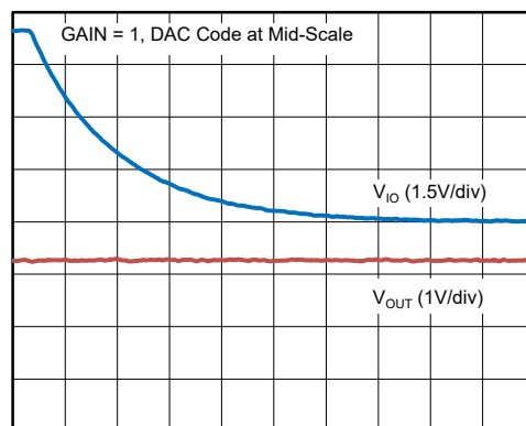
V_{IO} Power-Down
